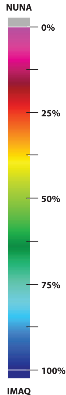
Titiraujaqsimajuq 1: Imaup Saqqijaarninganik Amiangata Utturautinga (%)
